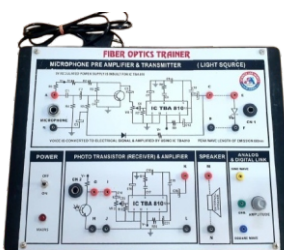
FIBER OPTICS TRAINER
